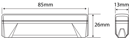
P/No. 85211A-R65 Amber shown not lit
